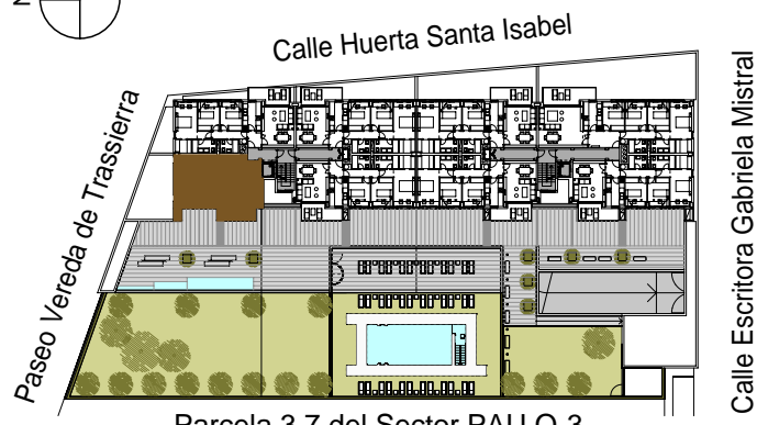
Parcela 3.7 del Sector PAU.O-3 UBICACION DE VIVIENDA EN EL EDIFICIO
